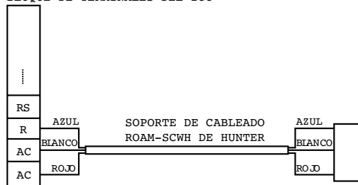
BLOQUE DE TERMINALES DEL ICC
